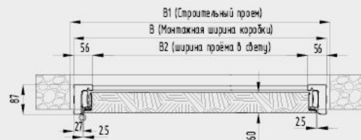
ДВЕРНАЯ КОРОБКА ДЛЯ ВРЕЗНОГО МОНТАЖА
